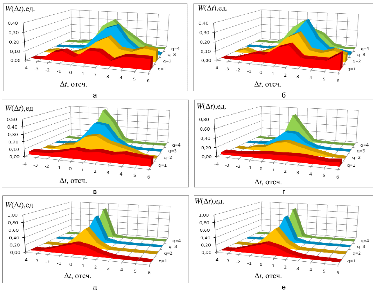
Рис. 6. Гистограммы W(\Delta t) значений ошибки оценивания положения максимума R-зубца QRS-комплекса электрокардиограммы корреляционно-экстремальным методом для: N=6, P_F = 0,05 (а); N=6, P_F = 0,01 (б); N=10, P_F = 0,05 (в); N=10, P_F = 0,01 (г); N=30, P_F = 0,05 (д); N=30, P_F = 0,01 (е) при частоте дискретизации 1000 Гц
