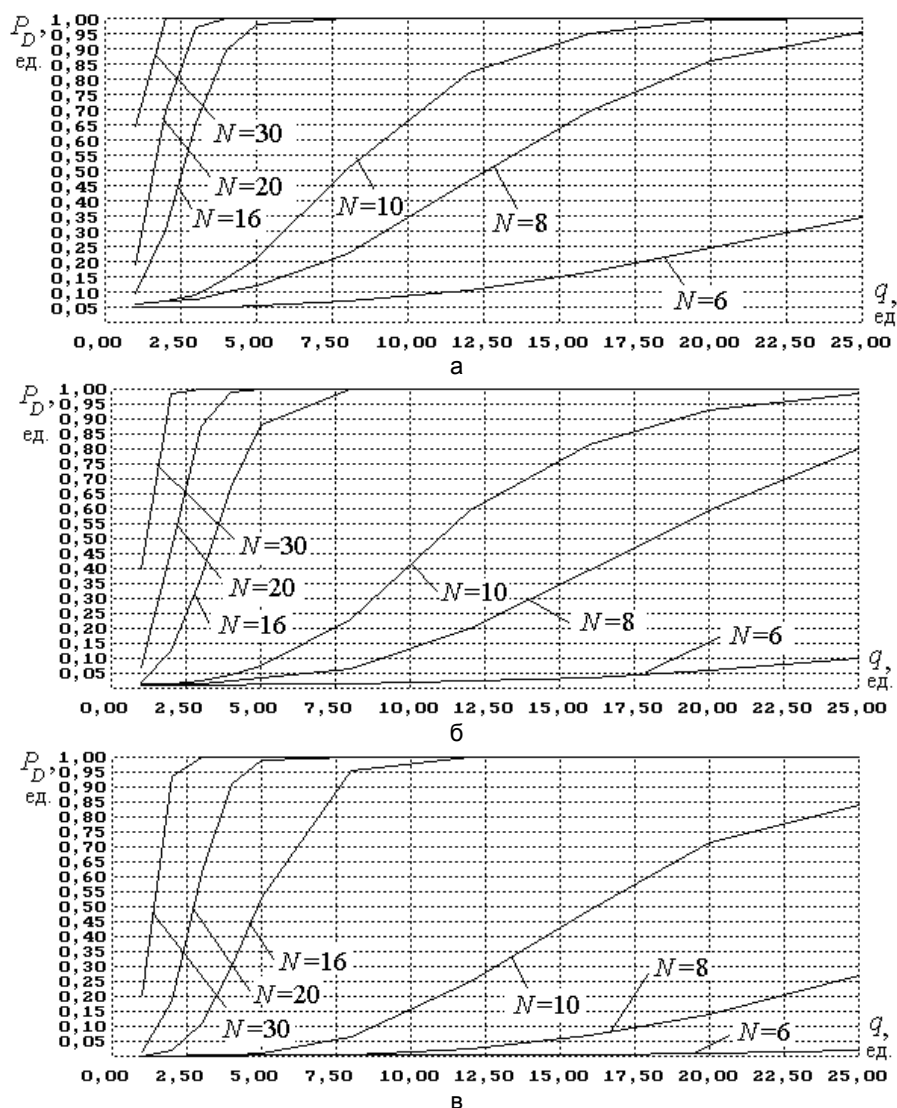
Рис. 5. Семейство характеристик обнаружения P_D(q) для корреляционно-экстремального метода обнаружения QRS-комплексов ЭКГ при различных значениях N и фиксированном значении P_F : для P_F = 0,05 (а); P_F = 0,01 (б); P_F = 0,001 (в)
