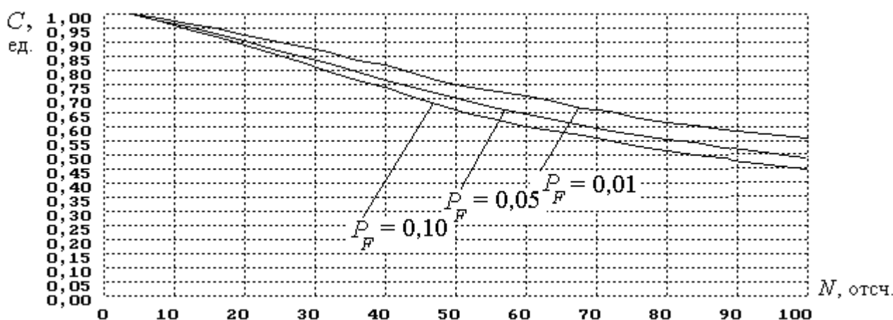
Рис. 4. Семейство зависимостей требуемого порогового уровня C для решающего правила алгоритма обнаружения ( \{k\} > C ) от числа отсчетов N и вероятности P_F
